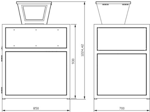
Fig. 4: L×W×H (mm) 可通过办公室门和电梯门
